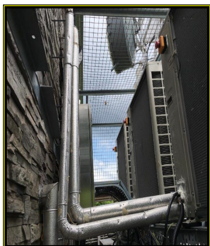
東平洲無線電發射站空氣調節機組
