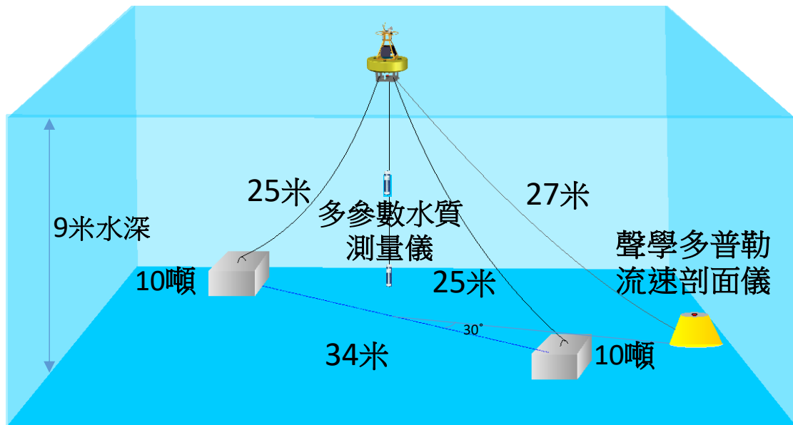
實時水文水質監測站示意圖
